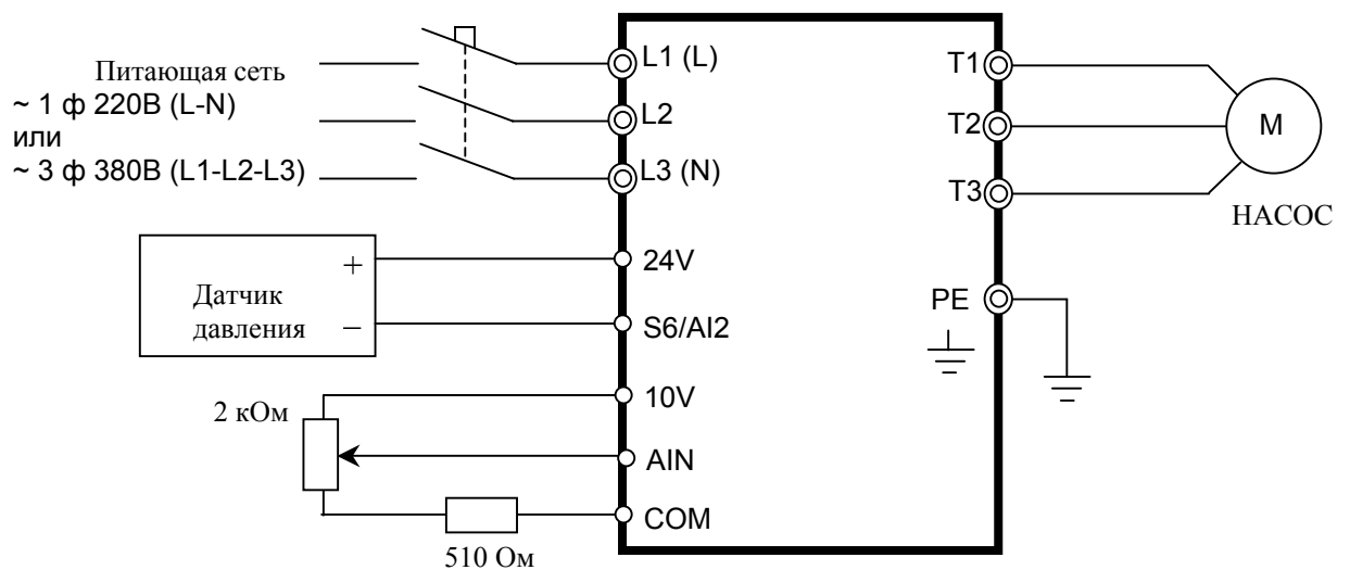
Пример. Управление насосом для поддержания заданного давления в системе (при произвольных изменениях расхода) с использованием преобразователя частоты и датчика давления. Схема подключения приведена на рисунке (применен датчик давления с токовым выходом 4-20 мА).
