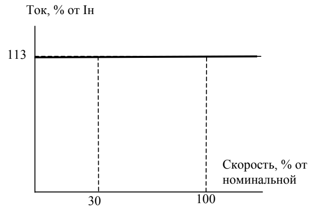
Вентиляторная нагрузка (9-10 = 1)
