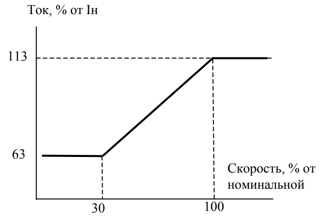
Вентиляторная нагрузка (9-10 = 1)
