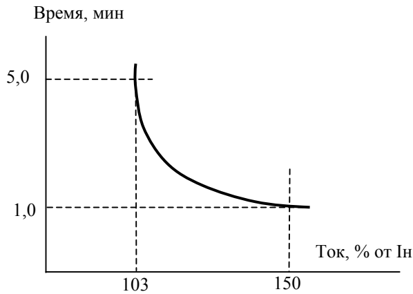
Нагрузка с постоянным моментом (9-10 = 0)
