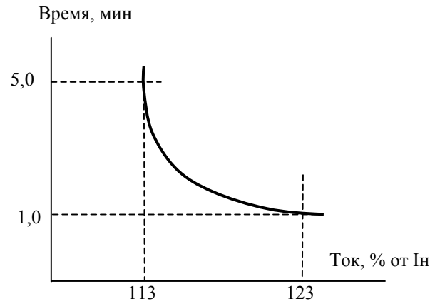
Вентиляторная нагрузка (9-10 = 1)
